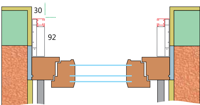
Shema montaže Mini Monoblock s pokrivnim vodilom
