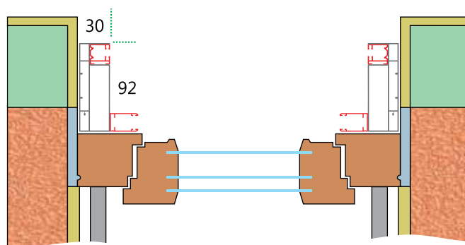
Shema montaže Mini Monoblock s komarnikom
