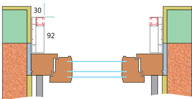
Shema montaže Mini Monoblock
