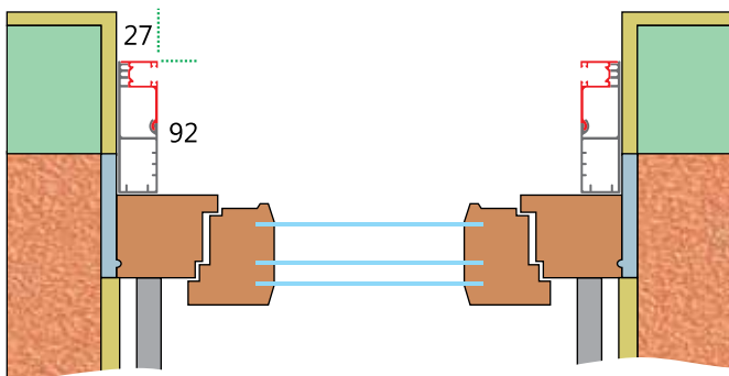
Shema montaže Compact vodilo (novo)
