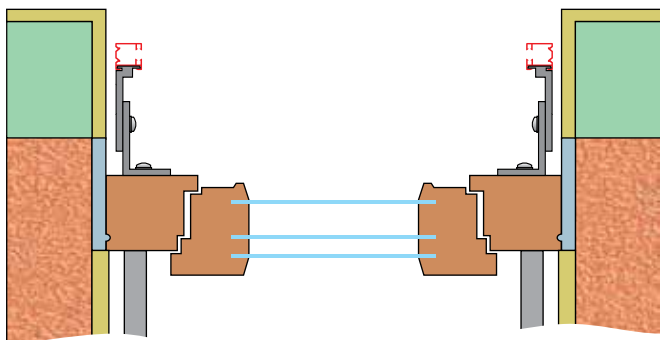
Shema montaže Z nastavljivim ALU nosilcem
