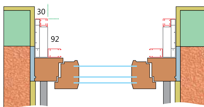
Shema montaže Mini Monoblock s pokrivnim vodilom in komarnikom
