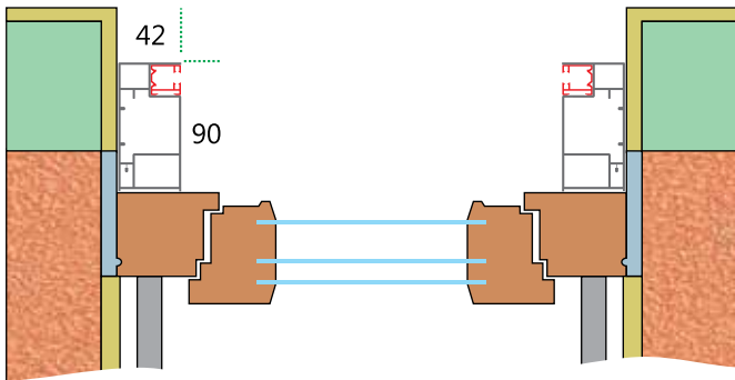
Shema montaže Monoblock
