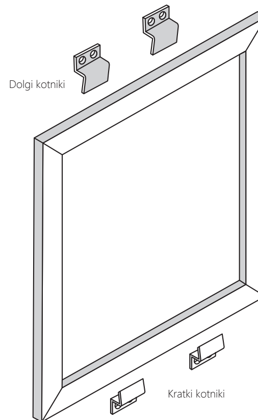
Prikaz pritrditve komarnika z držali
