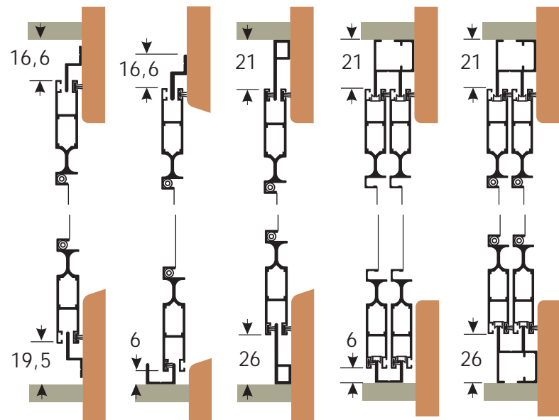
Prerezi montaže različnih profilov drsnega komarnika
