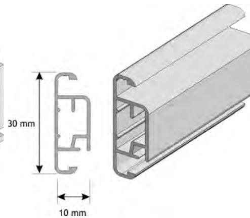
Prečni profil za večje komarnike
