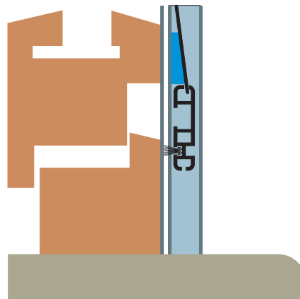
Standardno tesnenje s ščetko na okno (nastavljivo po višini).
