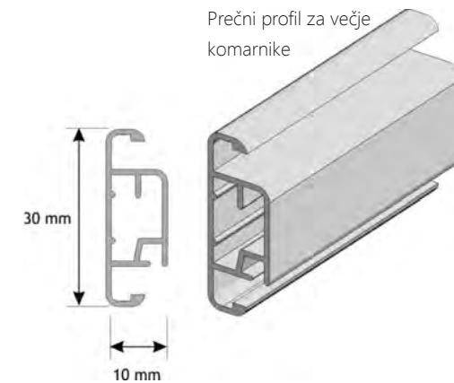
Fiksni profil z utorom za ščetko
