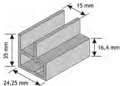
"2B" profil drsnega komarnika
