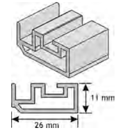
Prečni profil za večje komarnike
