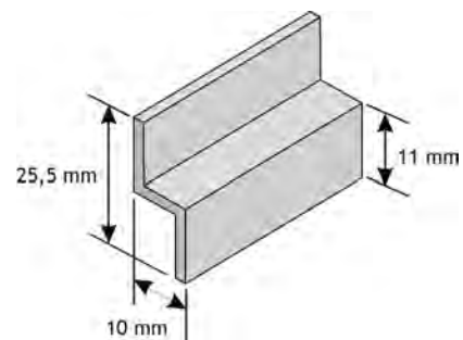
"Z" profil drsnega komarnika
