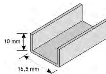
"U" profil drsnega komarnika
