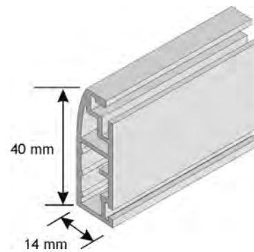
Profil okvirja vratnega komarnika
